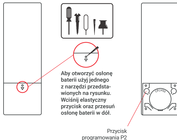
Nadajnik 1-kanalowy i 15-kanalowy (tył)
